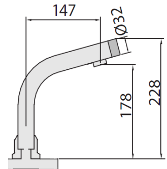
211-101/150-170/01 Berührungslose Multifunktionsarmatur, Tischmontage
